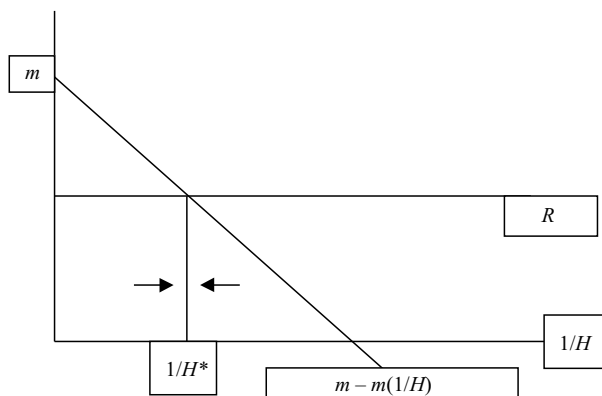
Figura 1 Diagrama de fase: a dinâmica do hiato tecnológico
